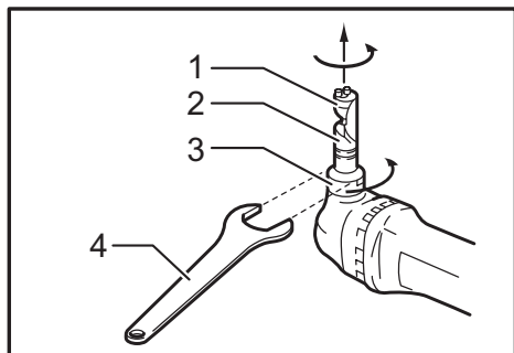
► 1. Die 2. Die holder 3. Lock nut 4. Wrench
